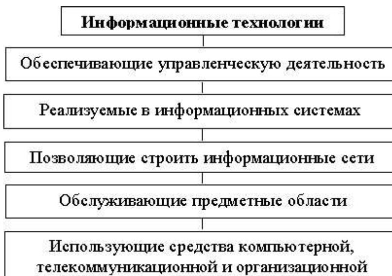
Рис. 3.1. Классификация ИТ.
